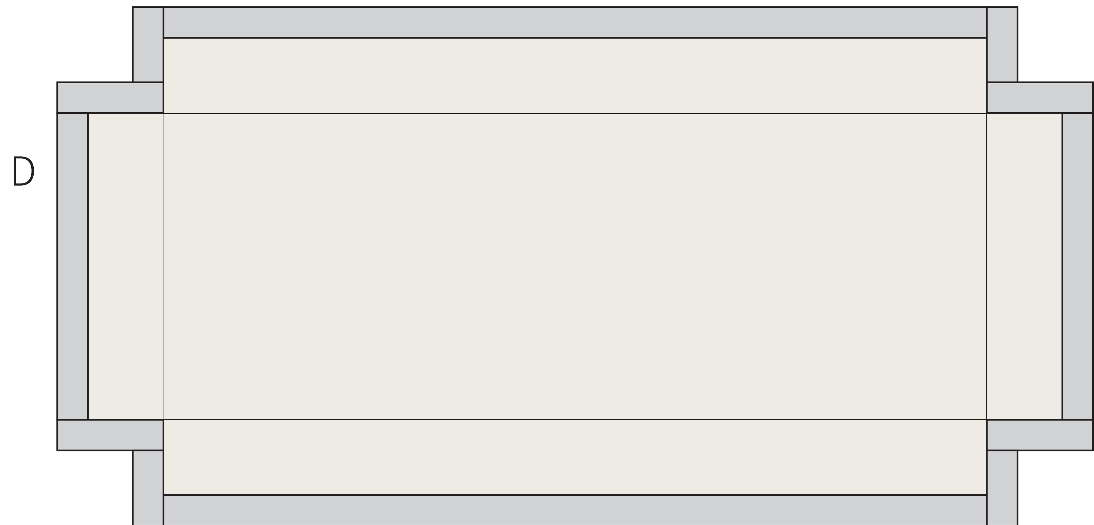
内盒裱纸: 尺寸:349X130X32mm
